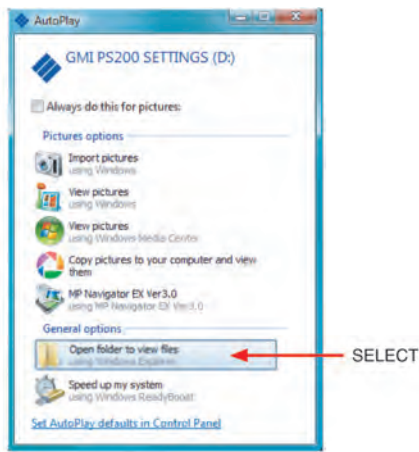
Fig. 3-2 Windows Vista™
